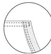
Figura 02 – Tecido aplicado na borda do bolso
